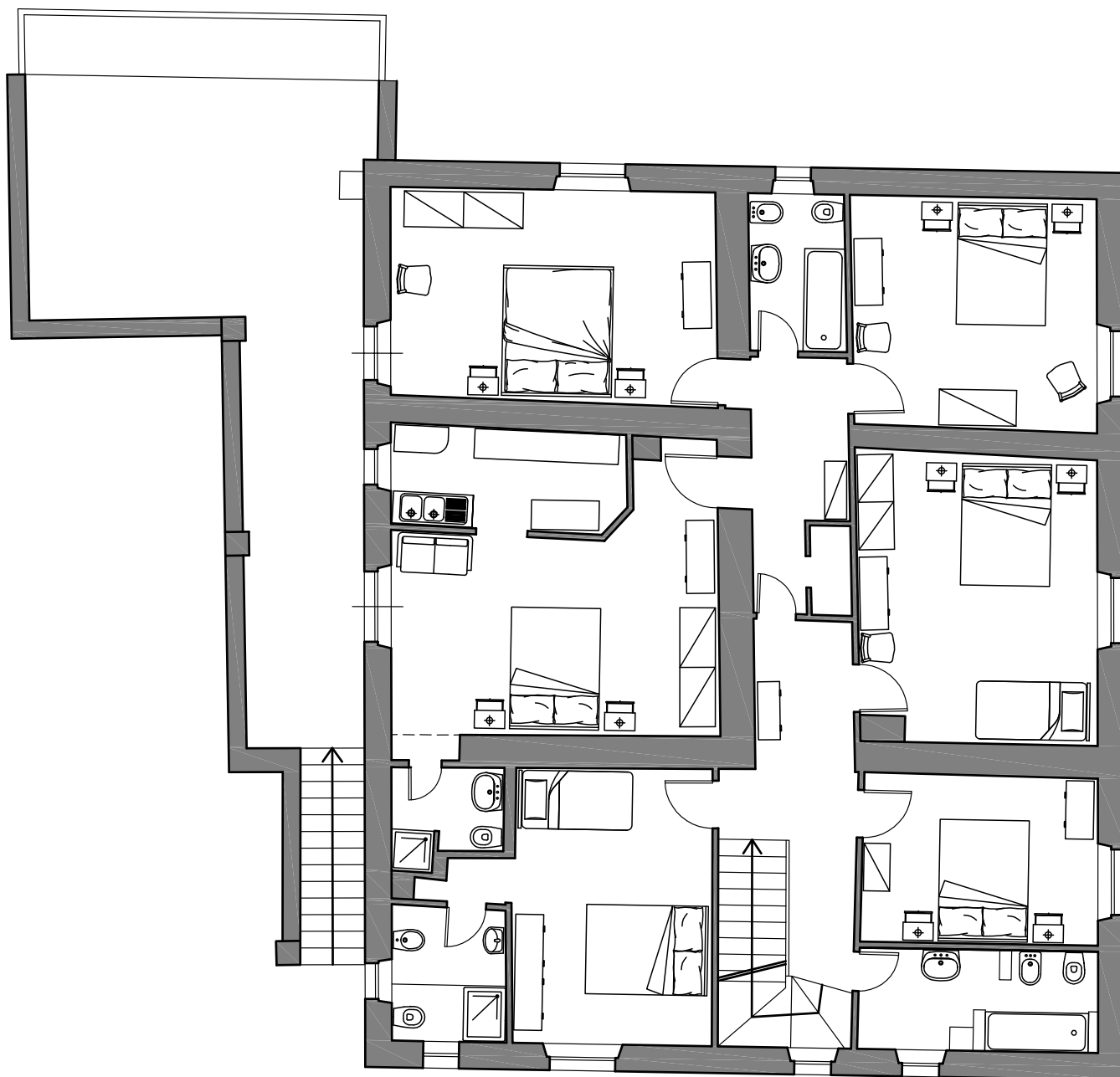
PIANO PRIMO
